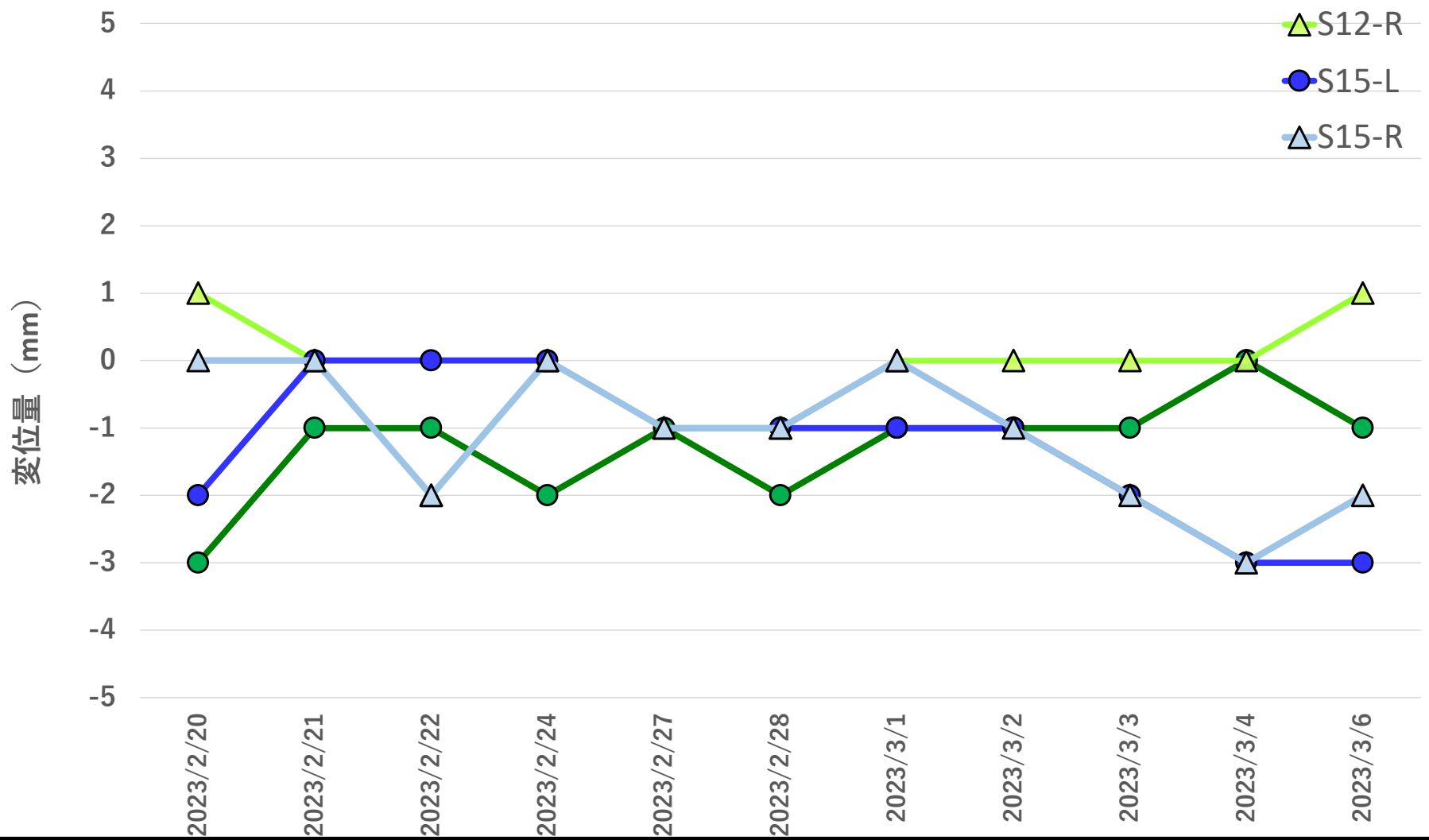
地盤変位量推移 2023年2月20日~2023年3月6日
