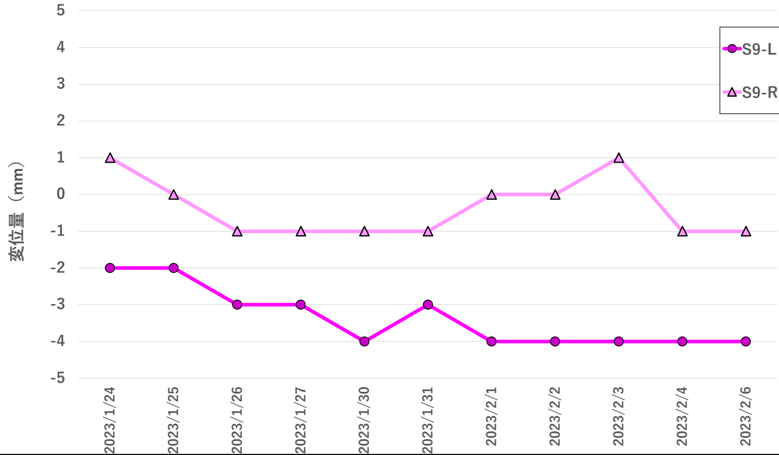
地盤変位量推移 2023年1月24日～2023年2月6日
