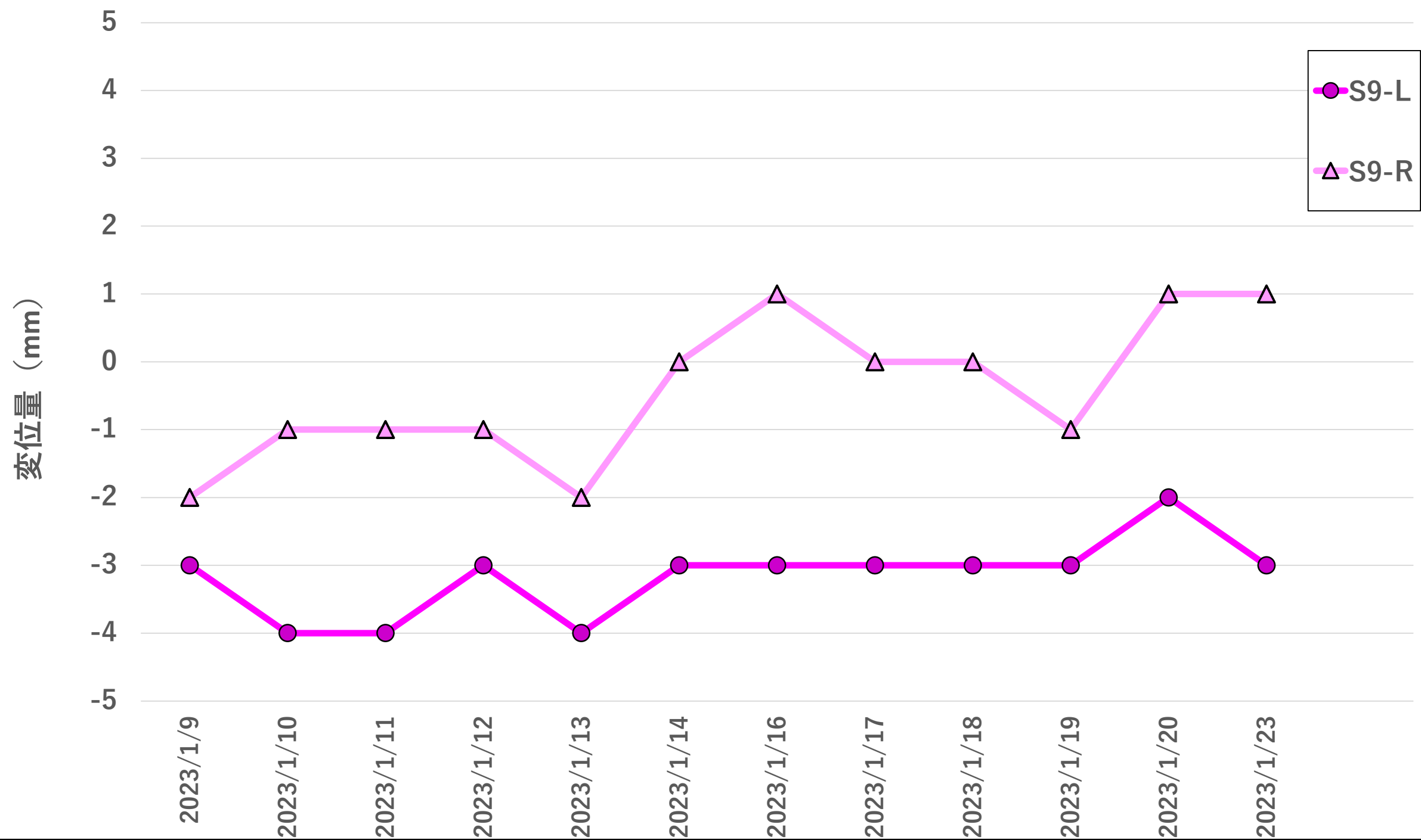
地盤変位量推移 2023年1月9日~2023年1月23日
