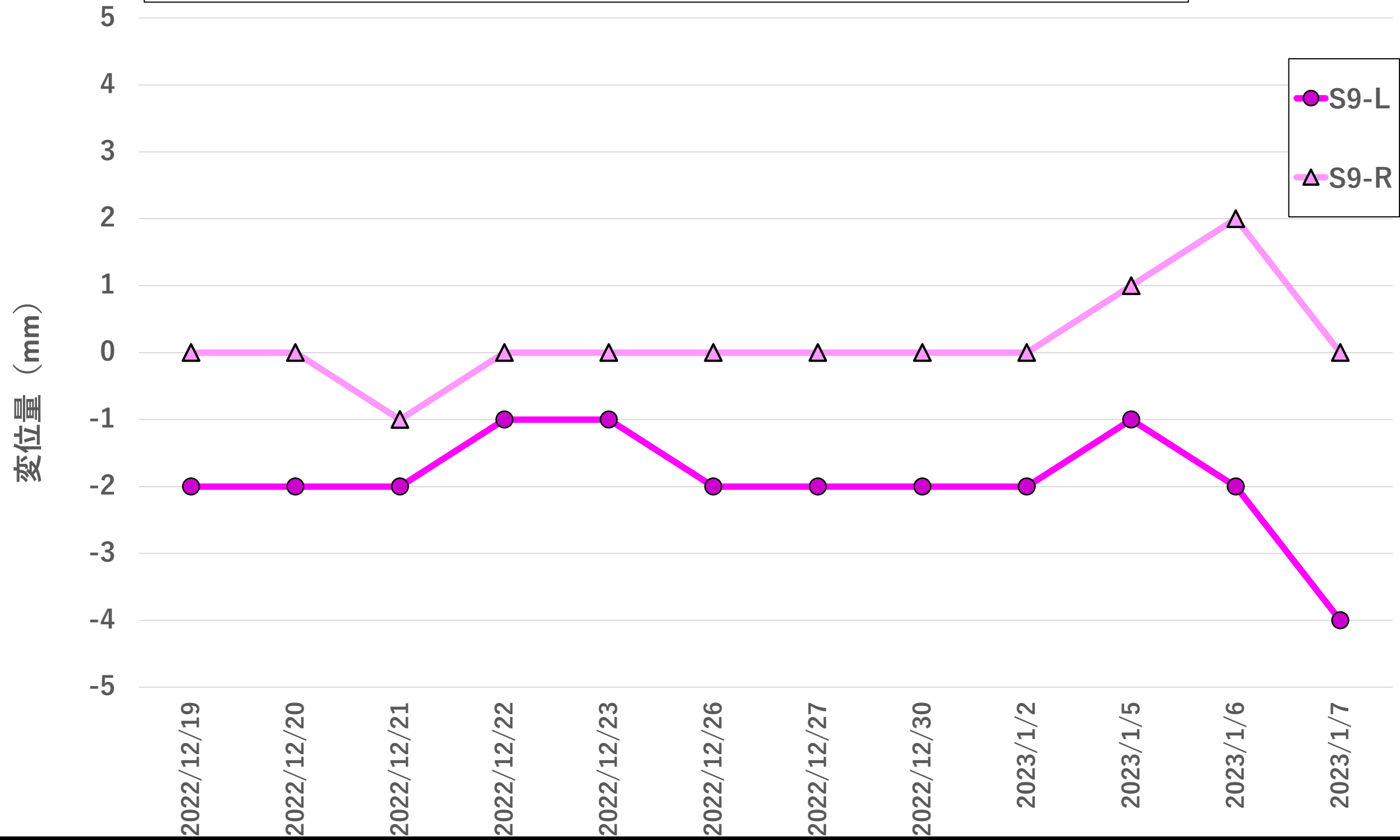
地盤変位量推移 2022年12月19日~2023年1月7日
