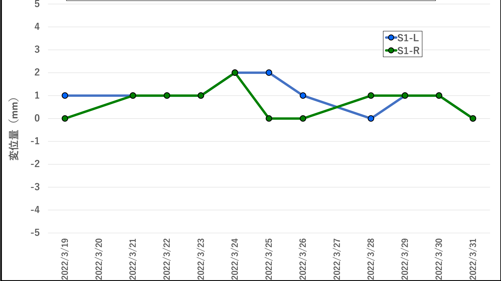
地盤変位量推移 2022年3月19日~2022年3月31日
